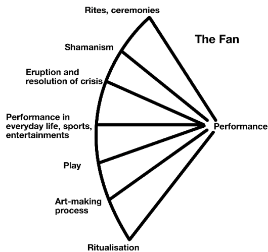
Figure 3: Schechner's Fan
